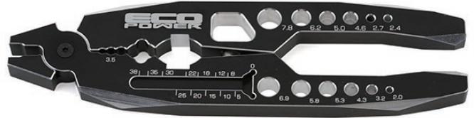
■ ECP-3057 EcoPower マルチファンクションショックシャフトプライヤー
